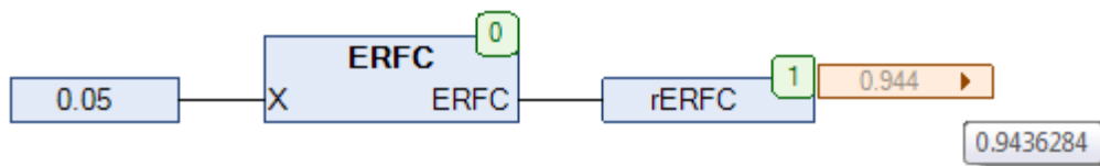
Рис. 5.42. Пример работы с функцией ERFC на языке CFC
