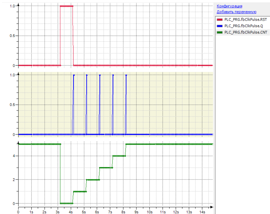
Рис. 15.15. Трассировка работы ФБ CLK_PULSE
