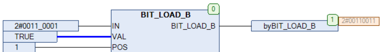
Рис. 16.6. Пример работы с функцией BIT_LOAD_B на языке CFC
