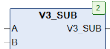
Рис. 11.19. Внешний вид функции V3_SUB на языке CFC
