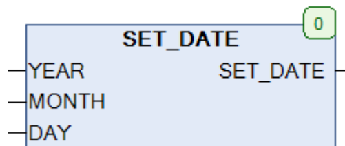
Рис. 12.88. Внешний вид функции SET_DATE на языке CFC
