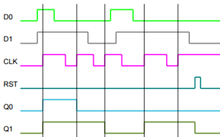
Рис. 17.5. Траассировка работы ФБ FF_D2E
