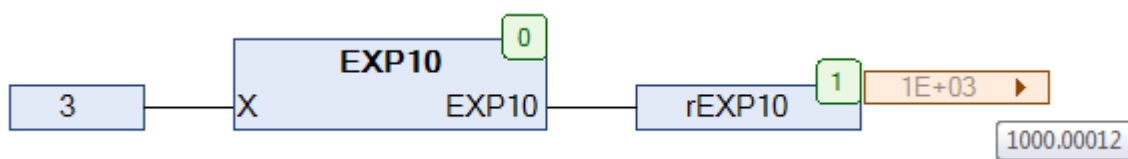
Рис. 5.46. Пример работы с функцией EXP10 на языке CFC
