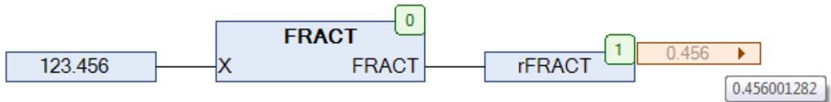
Рис. 5.58. Пример работы с функцией FRACT на языке CFC
