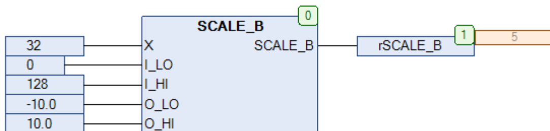
Рис. 19.47. Пример работы с функцией SCALE_B на языке CFC
