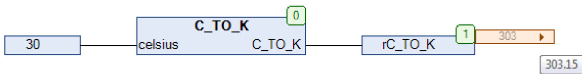
Рис. 22.9. Пример работы с функцией C_TO_K на языке CFC
