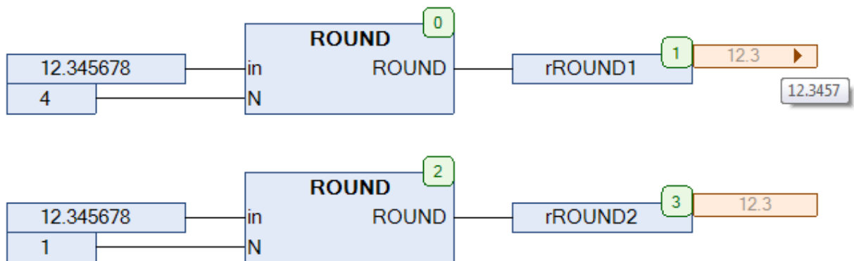
Рис. 5.112. Пример работы с функцией ROUND на языке CFC
