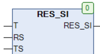
Рис. 20.9. Внешний вид функции RES_SI на языке CFC
