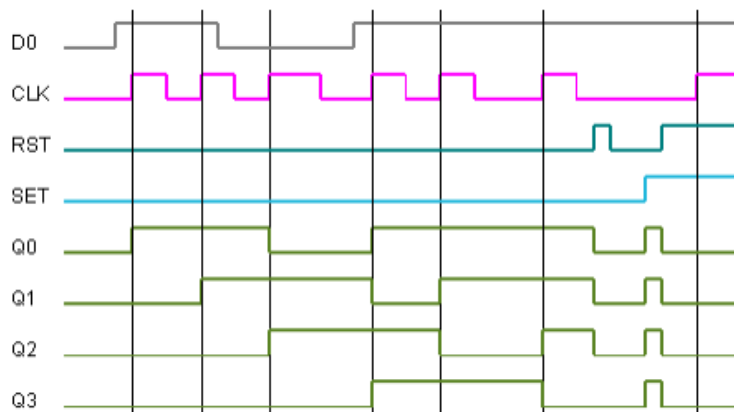
Рис. 17.15. Трассировка работы ФБ SHR_4E
