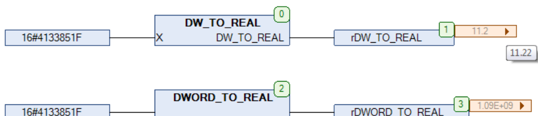
Рис. 16.46. Пример работы с функцией DW_TO_REAL на языке CFC
