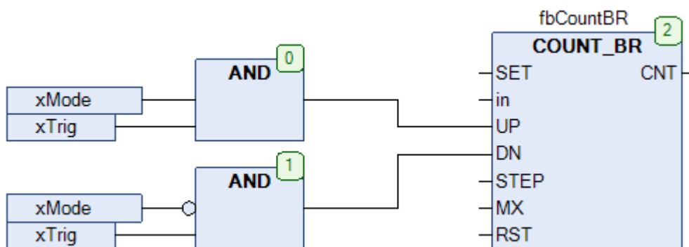
Рис. 17.2. Пример работы с ФБ COUNT_BR на языке CFC
