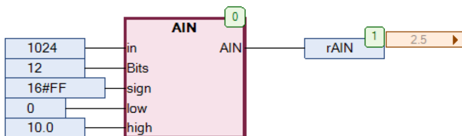
Рис. 19.2. Пример работы с функцией AIN на языке CFC
