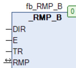
Рис. 18.1. Внешний вид ФБ _RMP_B на языке CFC
