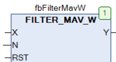
Рис. 19.23. Внешний вид ФБ FILTER_MAV_W на языке CFC
