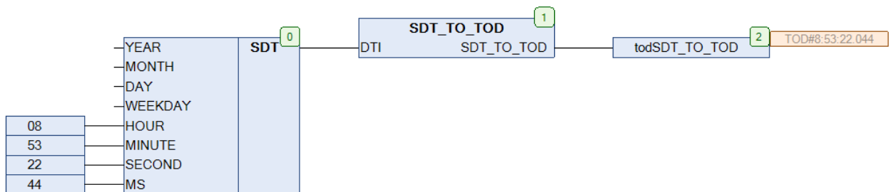
Рис. 12.81. Пример работы с функцией SDT_TO_TOD на языке CFC
