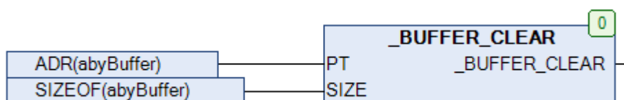
Рис. 25.1. Вызов функции работы с буфером на языке CFC
