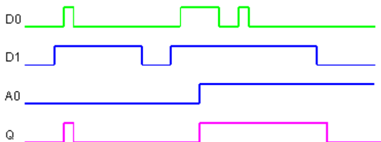
Рис. 16.59. Трассировка работы функции MUX_2
