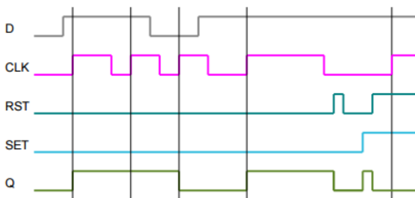
Рис. 17.10. Трассировка работы ФБ FF_JKE
