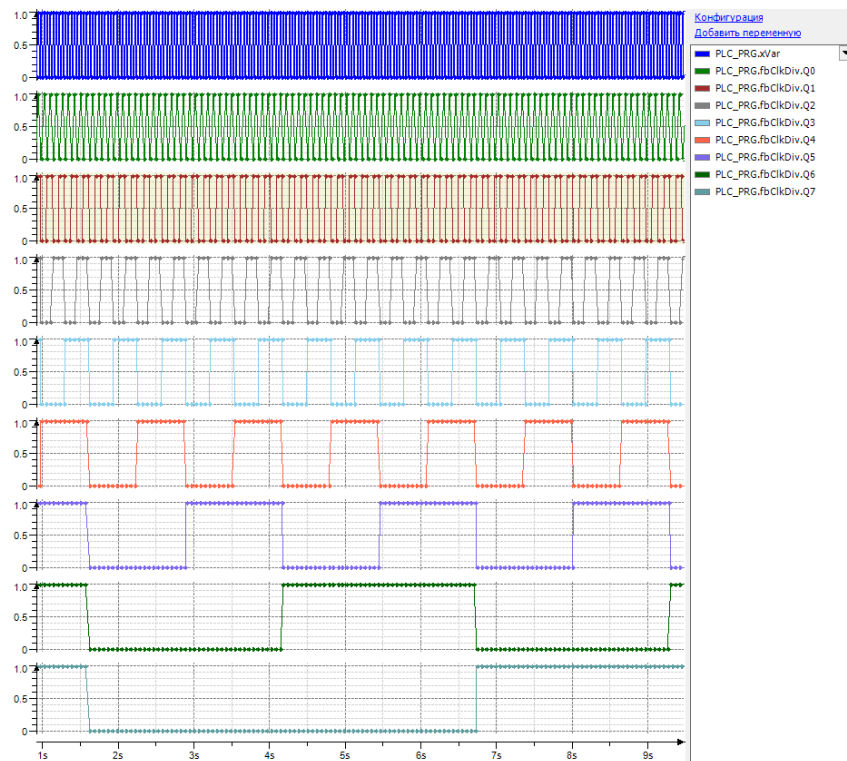
Рис. 15.9. Трассировка работы ФБ CLK_DIV
