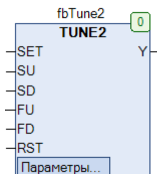
Рис. 24.26. Внешний вид ФБ TUNE2 на языке CFC
