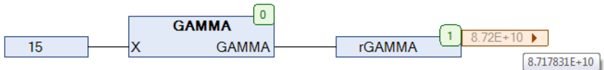
Рис. 5.60. Пример работы с функцией GAMMA на языке CFC
