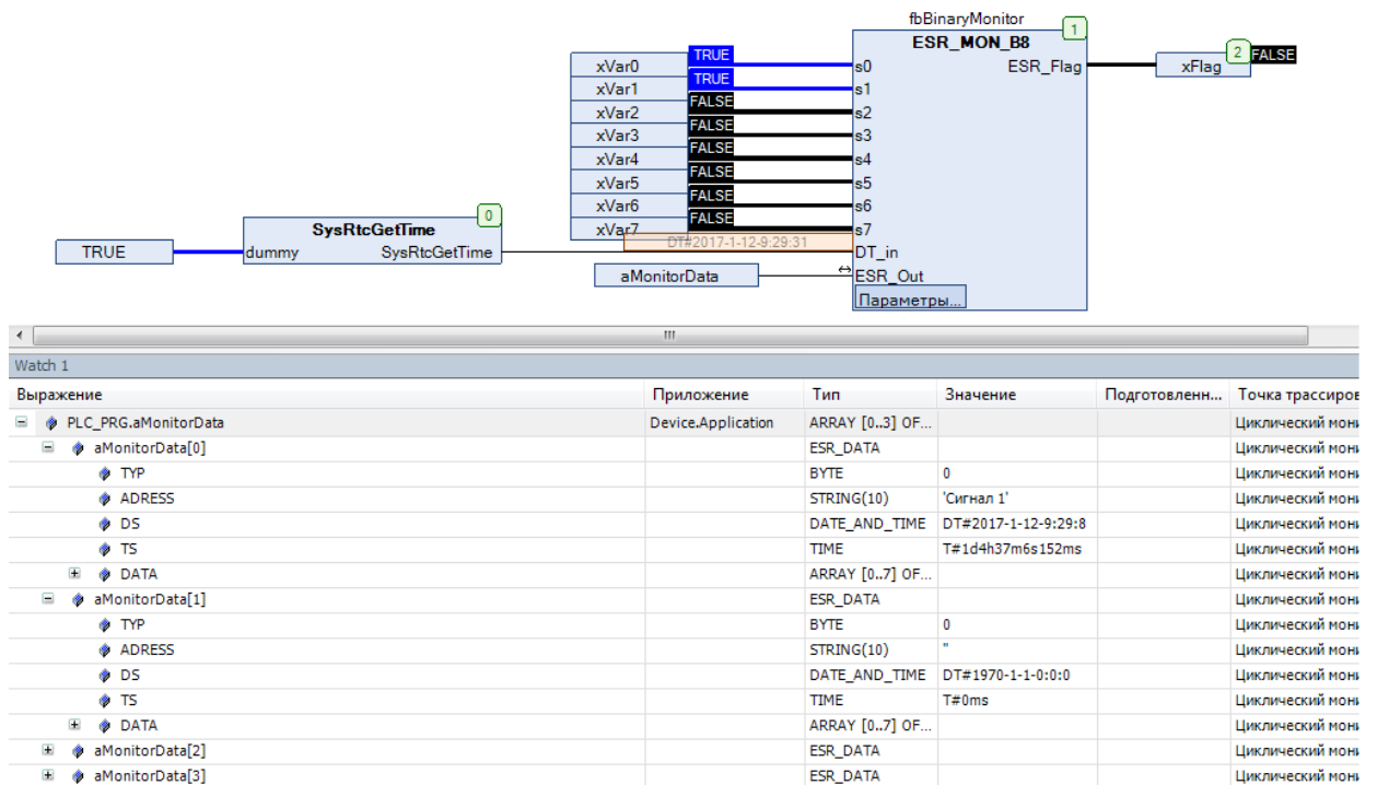
Рис. 4.6. Пример работы с ФБ ESR_MON_B8 на языке CFC. Спустя некоторое время изменился сигнал xVar1 ('Сигнал 1')
