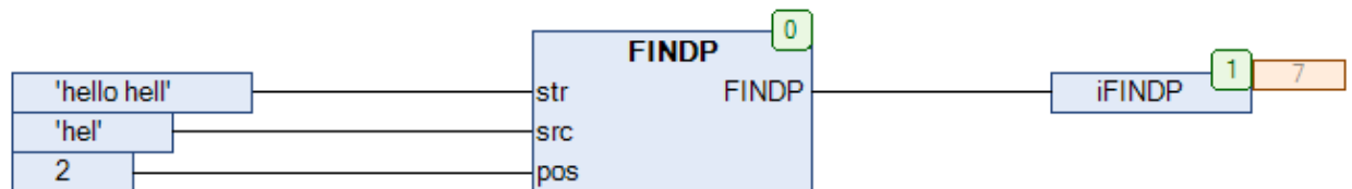
Рис. 13.58. Пример работы с функцией FINDP на языке CFC
