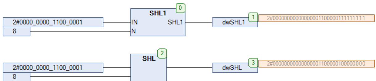
Рис. 16.73. Пример работы с функцией SHL1 на языке CFC
