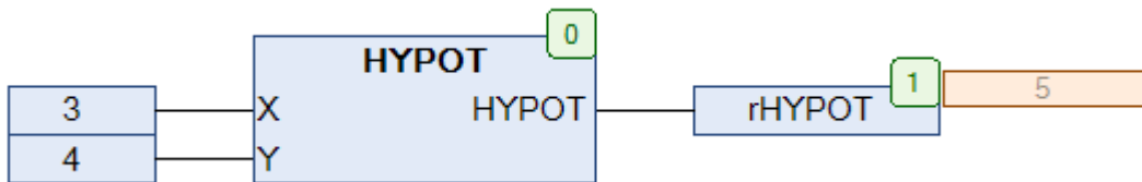
Рис. 5.72. Пример работы с функцией HYPOT на языке CFC
