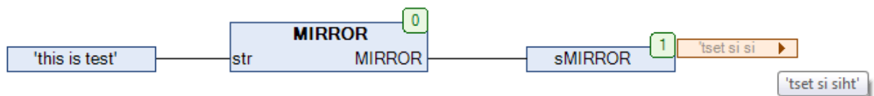
Рис. 13.116. Пример работы с функцией MIRROR на языке CFC
