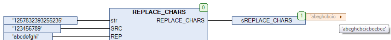
Рис. 13.128. Пример работы с функцией REPLACE_CHARS на языке CFC
