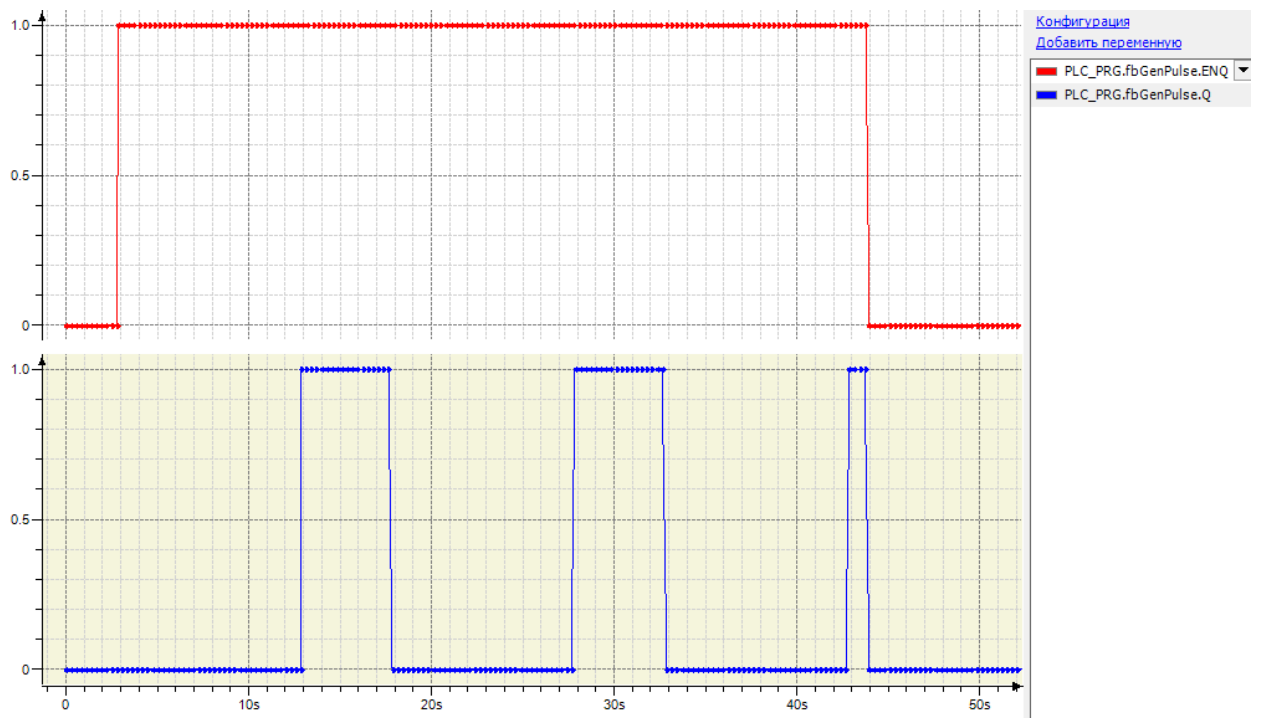
Рис. 18.7. Трассировка работы ФБ GEN_PULSE (РТН=Т#5s, РТЛ=Т#10s)
