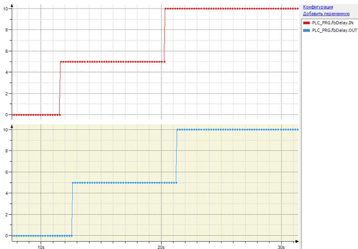
Рис. 19.12. Трассировка работы ФБ DELAY для ПЛК с временем цикла=100 мс, N=10
