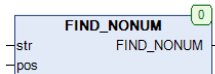
Рис. 13.47. Внешний вид функции FIND_NONUM на языке CFC
