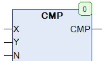
Рис. 5.25. Внешний вид функции CMP на языке CFC
