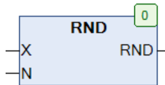
Рис. 5.109. Внешний вид функции RND на языке CFC
