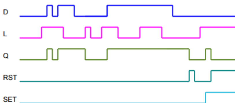
Рис. 17.13. Трассировка работы ФБ LTCH
