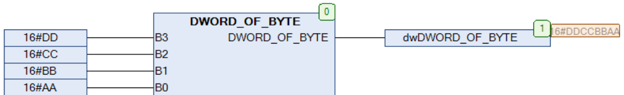
Рис. 16.48. Пример работы с функцией DWORD_OF_BYTE на языке CFC
