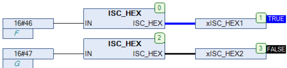
Рис. 13.102. Пример работы с функцией ISC_HEX на языке CFC
