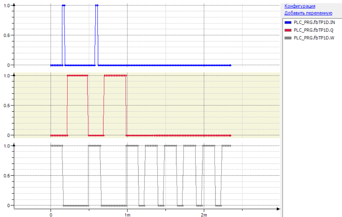
Рис. 15.43. Трассировка работы ФБ TP_1D
