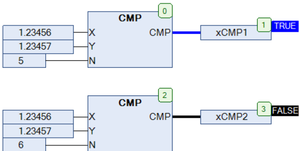
Рис. 5.26. Пример работы с функцией CMP на языке CFC
