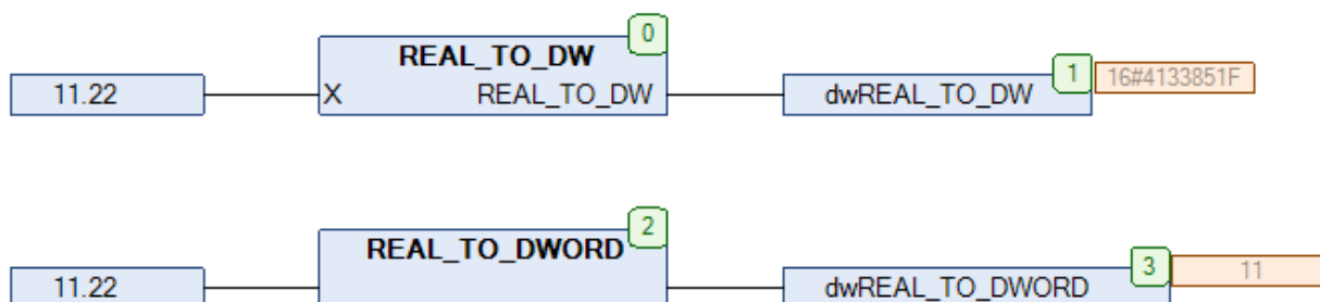
Рис. 16.67. Пример работы с функцией REAL_TO_DW на языке CFC
