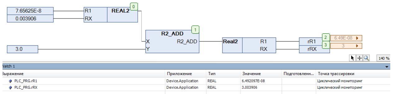
Рис. 8.4. Пример работы с функцией R2_ADD на языке CFC
