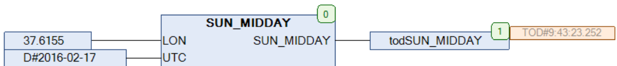
Рис. 12.95. Пример работы с функцией SUN_MIDDAY на языке CFC
