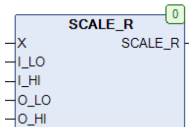
Рис. 19.54. Внешний вид функции SCALE_R на языке CFC
