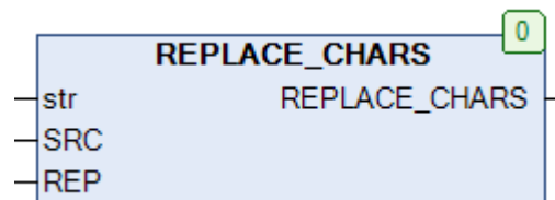
Рис. 13.127. Внешний вид функции REPLACE_CHARS на языке CFC
