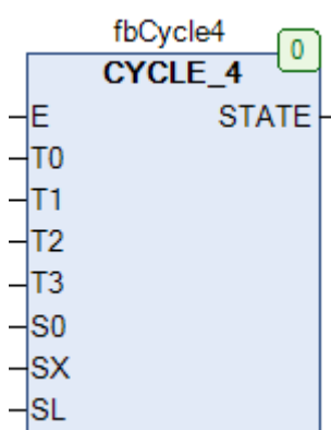
Рис. 15.16. Внешний вид ФБ CYCLE_4 на языке CFC
