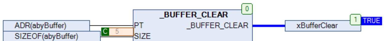
Рис. 25.3. Пример работы с функцией _BUFFER_CLEAR на языке CFC
