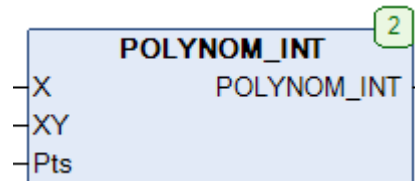
Рис. 9.21. Внешний вид функции POLYNOM_INT на языке CFC
