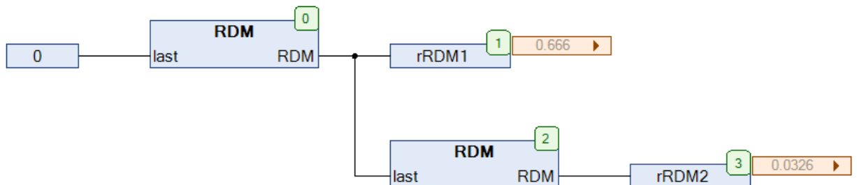
Рис. 5.100. Пример работы с функцией RDM на языке CFC
