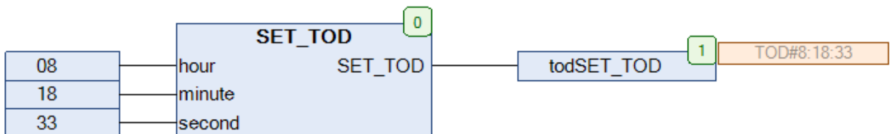
Рис. 12.93. Пример работы с функцией SET_TOD на языке CFC
