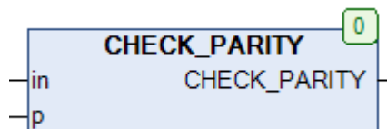
Рис. 16.35. Внешний вид функции CHECK_PARITY на языке CFC
