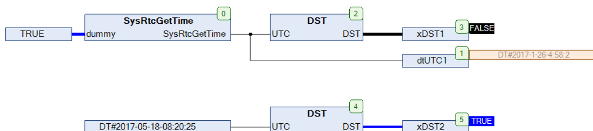
Рис. 12.23. Пример работы с функцией DST на языке CFC
