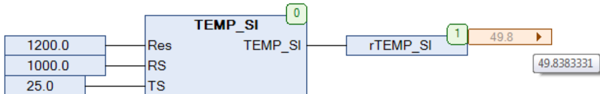
Рис. 20.20. Пример работы с функцией TEMP_SI на языке CFC (для ТС KTY83 )
