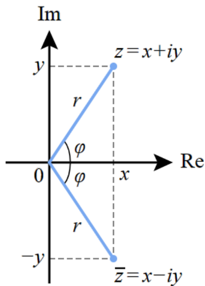
Рис. 7.22. Геометрическое представление сопряженных чисел
