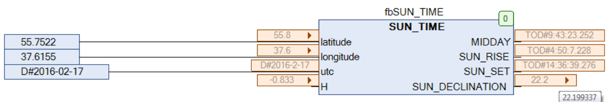
Рис. 12.99. Пример работы с ФБ SUN_TIME на языке CFC
