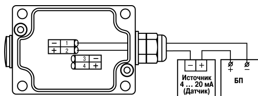
Рисунок 4 – Подключение справа
