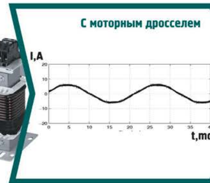
Моторный дроссель
