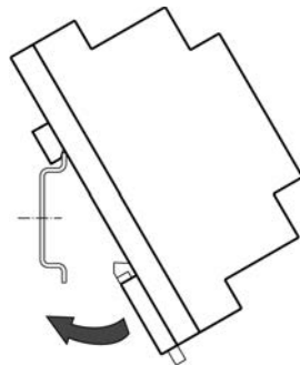
Рисунок 5.3 – Монтаж прибора с креплением на DIN-рееку
