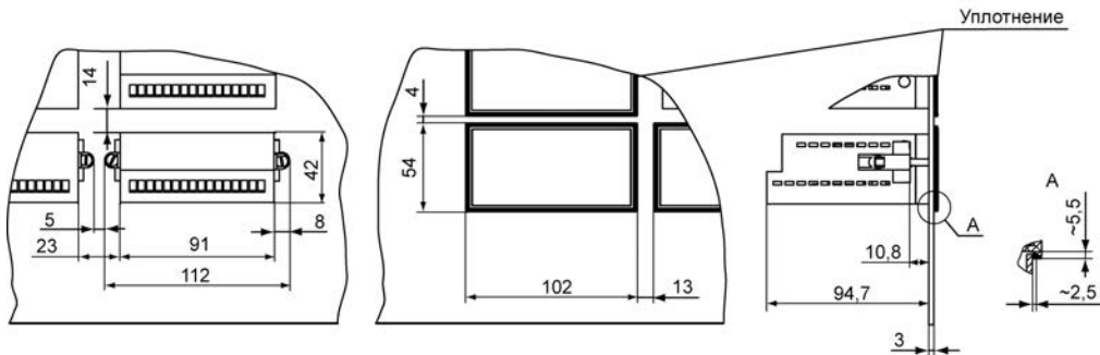
Рисунок А.7 - Прибор в корпусе Щ2, установленный в щит толщиной 3 мм
