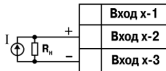
Рис. Б.4. Схема подключения активного датчика с токовым выходом 0 ... 5, 0 ... 20 или 4 ... 20 мА
