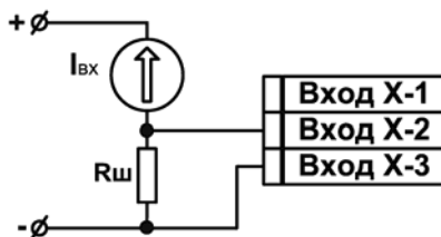
Рисунок Б.5 – Схема подключения активного датчика с токовым выходом 0... 5, 0... 20 или 4...20 мА
