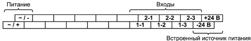
Рисунок Б.1 – Клеммная колодка прибора
