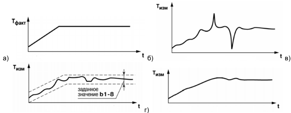
Рисунок 3.2 – Временные диаграммы работы цифрового фильтра: контролируемая температура (а), фильтры отключены (б), включен фильтр b1-8 (в), включены фильтры b1-8 и b1-9 (г)
