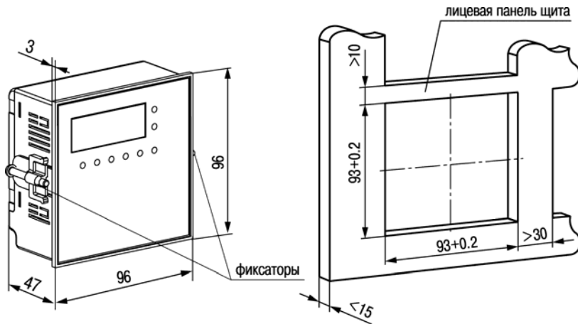
Рисунок А.1 – Габаритный и установочный чертеж прибора
