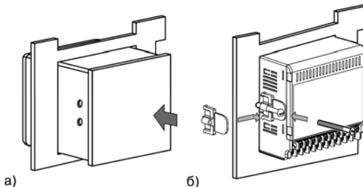
Рисунок 5.1 – Установка приборов щитового исполнения
