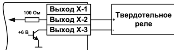
Рисунок Б.8 – Схема подключения нагрузки к ВУ типа Т
