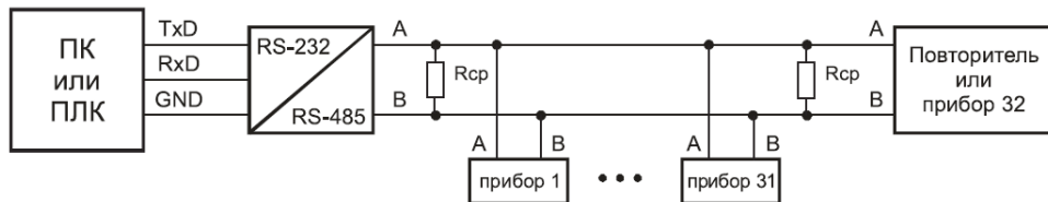
Рис. 1.1. Типовая схема промышленной сети RS-485
