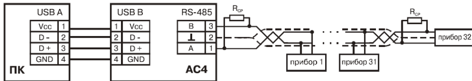
Рис. 6.1. Схема подключения прибора AC4
