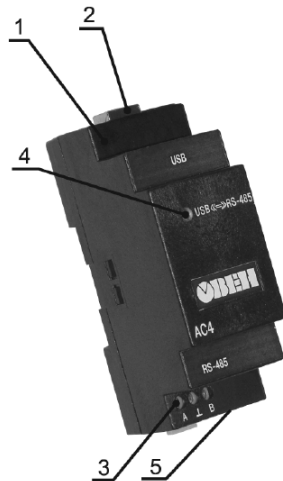
Рис. 4.1. Внешний вид прибора AC4
