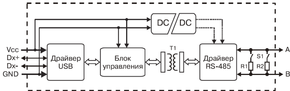
Рис. 4.2. Функциональная схема прибора AC4
