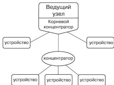
Рисунок 1.2 – Топология физической шины USB
