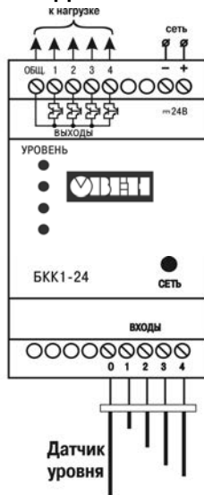
Рисунок Б.1 – Схема подключения БКК1-24
