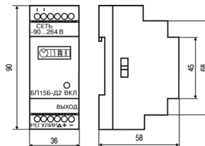
Рисунок 4.1 – Габаритные размеры блока питания БП15Б-Д2-х
