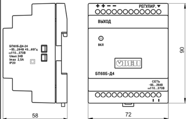
Рисунок 3.1 – Габаритные размеры блока
