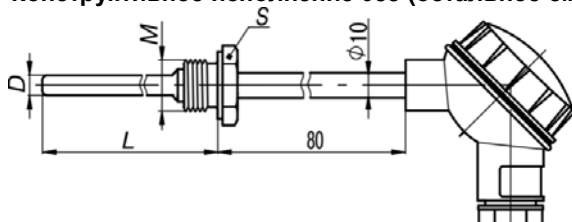
Рисунок А.4 – Конструктивное исполнение 065, 075 и 085
