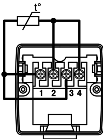
в) четырехпроводная
