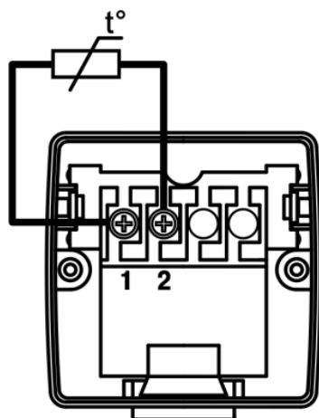
а) двухпроводная
