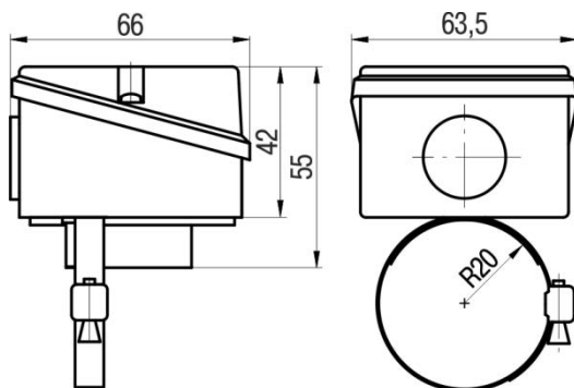
Рисунок Г.5 – Конструктивное исполнение 3005
