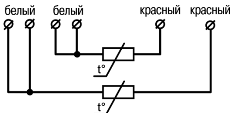
б) трехпроводная
