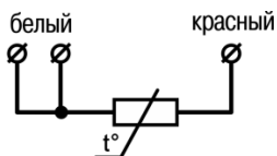
б) трехпроводная
