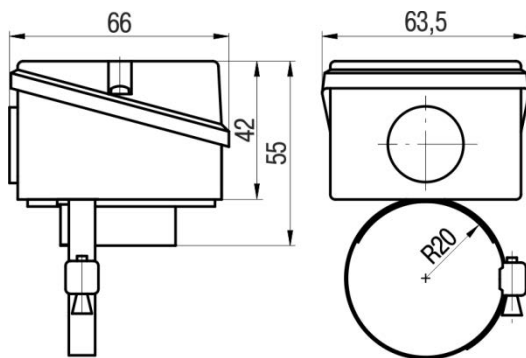
Рисунок Г.5 – Конструктивное исполнение 3225
