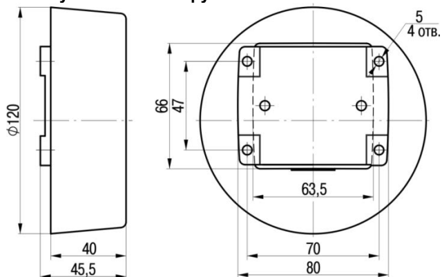
Рисунок Г.6– Конструктивное исполнение 3005
