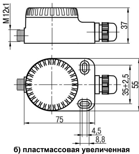
Рисунок В.3 – Конструктивные исполнения коммутационных головок для ДТС 125
