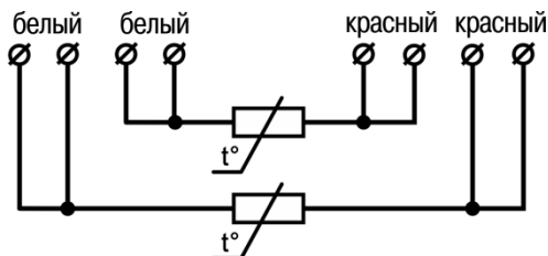
в) четырехпроводная
