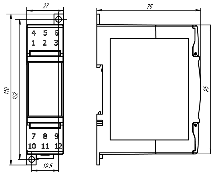
Рисунок А.1 – Габаритный чертеж барьера
