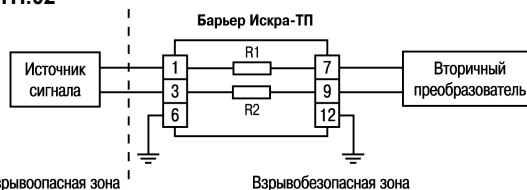
Рисунок 3.2 – Схема подключения барьера, R1=R2=110 \text{ Ом} \pm 5 \%
