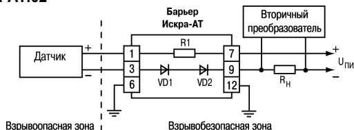
Рисунок 3.1 – Схема подключения барьера, R1=390 \text{ Ом} \pm 5 \% ; VD1, VD2 – диоды КД208
