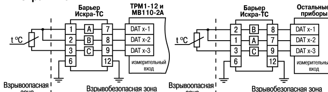
Рисунок 3.3 – Схема подключения барьера
