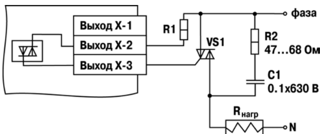
Рисунок 5.2 - Схема подключения оптосимистора
