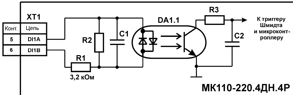
Рисунок Б.7 – Электрическая принципиальная схема дискретного входа МК110-220.4ДН.4Р (схема других входов идентична приведенной)
