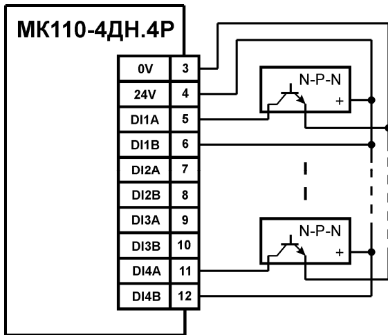
Рисунок Б.4 – Схема подключения к МК110-220.4ДН.4Р дискретных датчиков с транзисторным выходом n-p-n-типа с ОК
