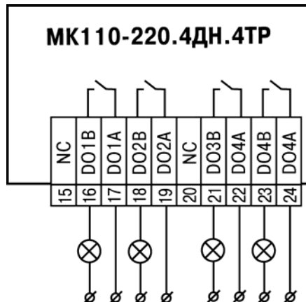
Рисунок Д.1 - Проверка выходов типа ТР
