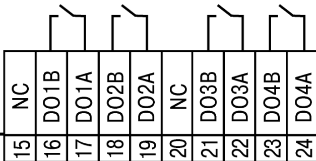
Рисунок Б.2 - Схема подключения к ВЭ типа твердотельное реле
