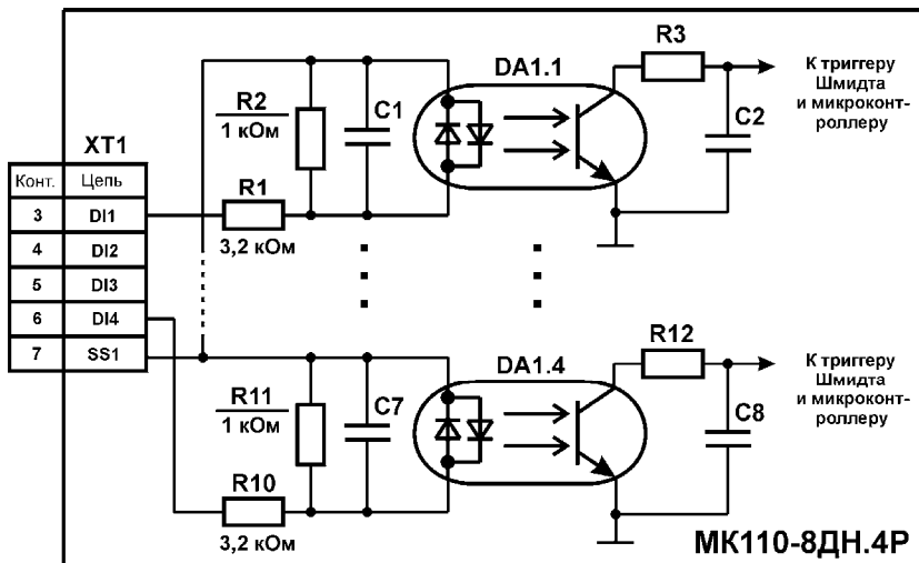
Рисунок Б.9 – Электрическая принципиальная схема группы дискретных входов МК110-8ДН.4Р (схема других групп входов идентична приведенной)
