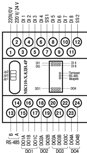
Рисунок Б.1 – Общий чертеж МК110
