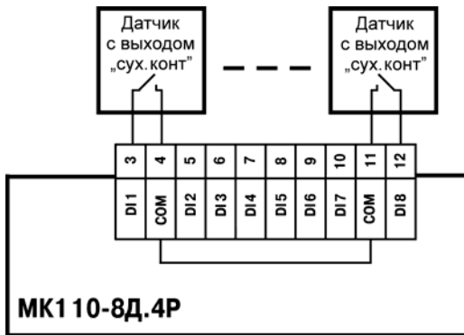
Рисунок Б.3 – Схема подключения к МК110-8Д.4Р дискретных датчиков с выходом типа «сухой контакт»
