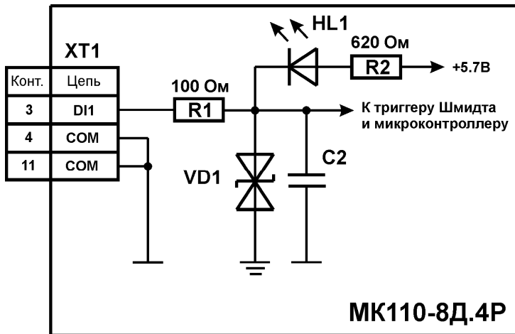
Рисунок Б.8 – Электрическая принципиальная схема входа МК110-8Д.4Р (схема других входов идентична приведенной)
