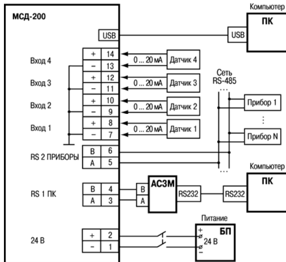
Рисунок Б.1 – Подключение к модулю внешних устройств
