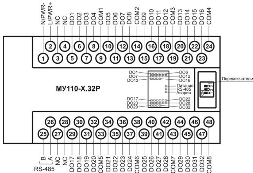
Рисунок Б.1 – Общий чертеж MY110-32P
