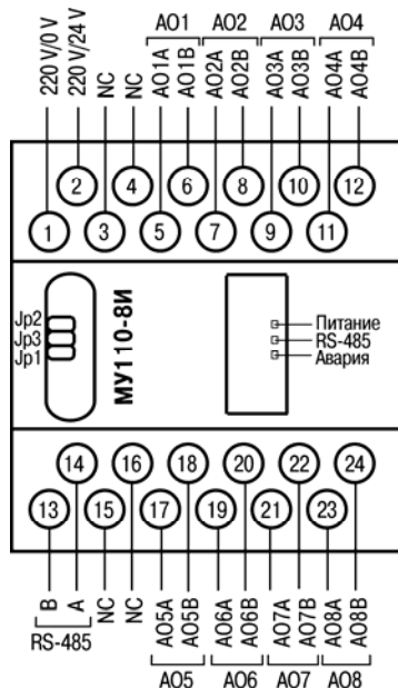
Рисунок Б.1 - Общий чертеж МУ110-8И
