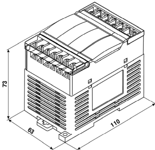
Рисунок А.1 - Габаритный чертеж МУ110-8И
