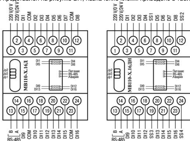
Рисунок Б.1 - Общий чертеж MB110-16Д(ДН)
