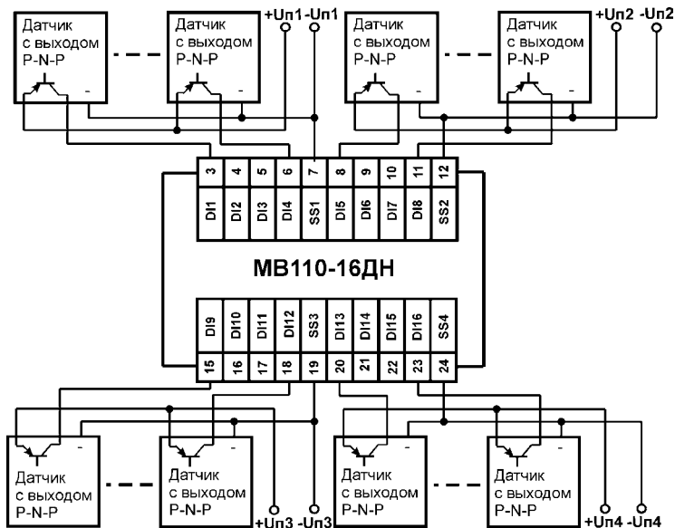
Рисунок Б.6 - Схема подключения к МВ110-16ДН дискретных датчиков с транзисторным выходом р-п-р-типа
