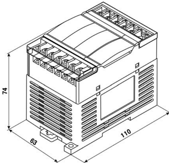
Рисунок А.1 – Габаритный чертеж прибора
