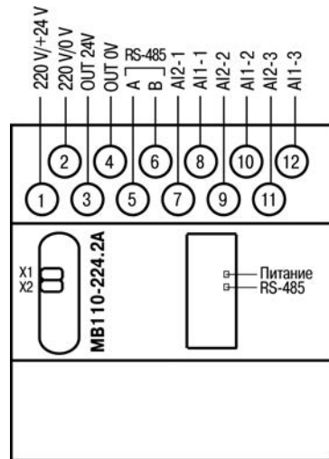
Рисунок Б.1 - Общий чертеж MB110-2A
