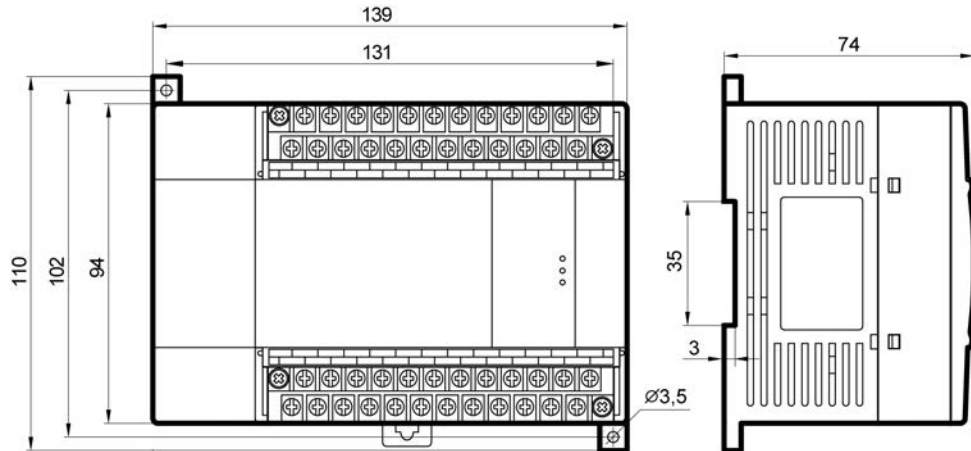
Рисунок А.1 – Габаритно-установочный чертеж MB110
