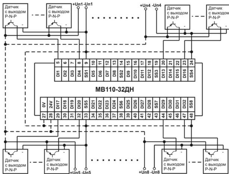
Рисунок Б.4 – Схема подключения к MB110-32ДН дискретных датчиков с транзисторным выходом р-п-р-типа
