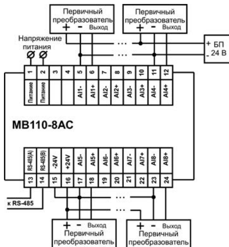
Рисунок Б.3 – Подключение к прибору трехпроводных первичных преобразователей
