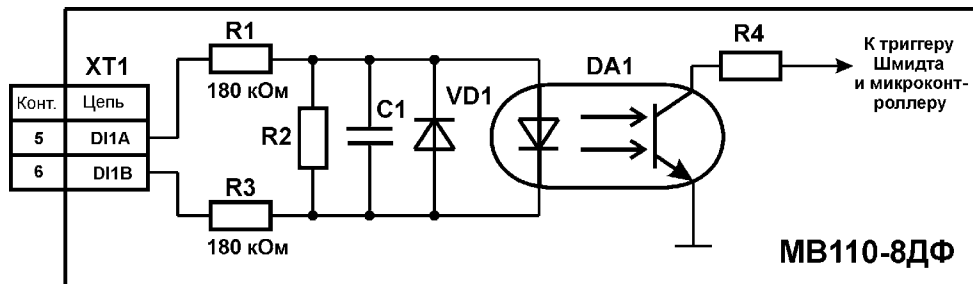
Рисунок Б.5 - Электрическая принципиальная схема входа MB110-8ДФ (схема других входов идентична приведенной)
