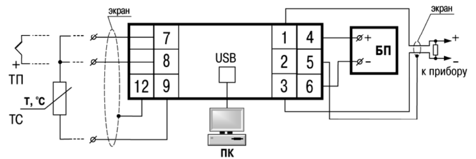
Рисунок 3 – Клеммные соединители преобразователя и схема подключения датчиков
