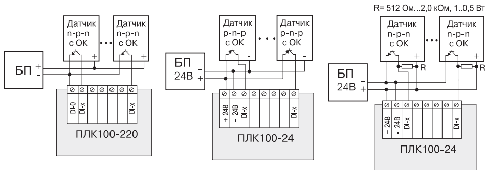
Рисунок Б.8 - Схемы подключения к ПЛК100 дискретных датчиков с полупроводниковым выходным каскадом: а – ПЛК100-220 датчик п-р-п-типа, б – ПЛК100-24 датчик р-п-р-типа, в – ПЛК100-24 датчик п-р-п-типа
