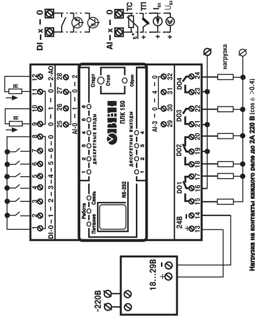
Рисунок Б.1 - Схема подключения питания, входов и выходов к ПЛК150-24.X-X
