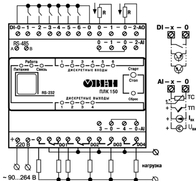
Рисунок Б.2 - Схема подключения питания, входов и выходов к ПЛК150-220.X-X
