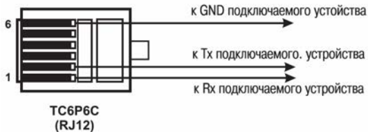
Рисунок Б.5 - Схема кабеля для подключения к порту Debug RS-232
