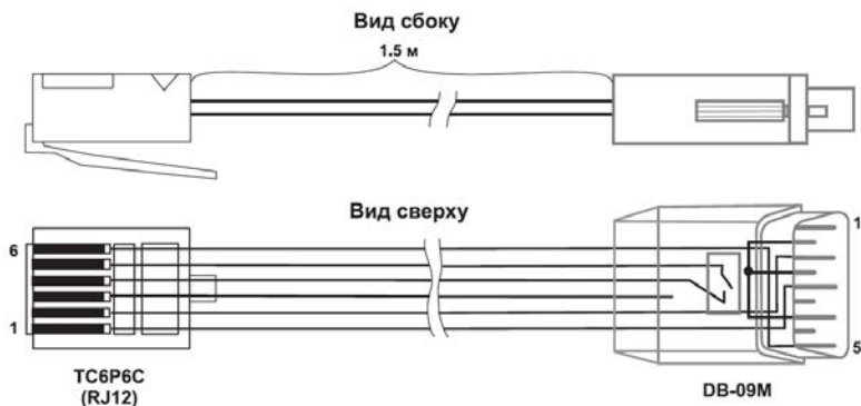
Рисунок Б.4 - Схема "Модемный кабель ПЛК1XX"
