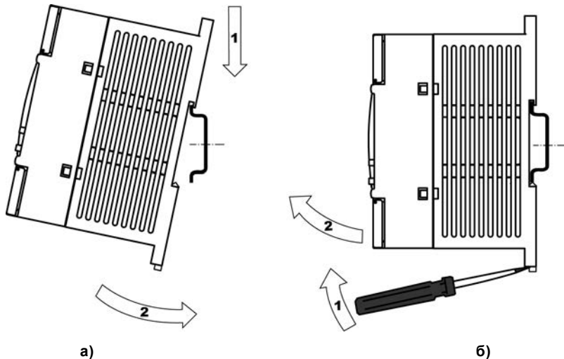
а) б) Рисунок 6.1 – Монтаж контроллера с креплением на DIN-рейку
