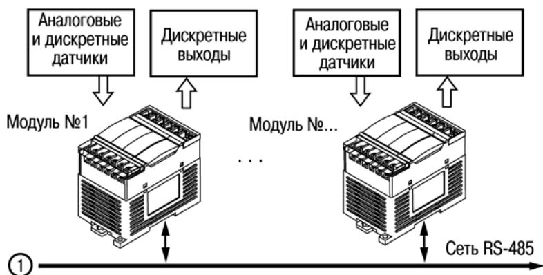
Рисунок 6.4 – Пример структуры соединений при использования ПЛК в системе
