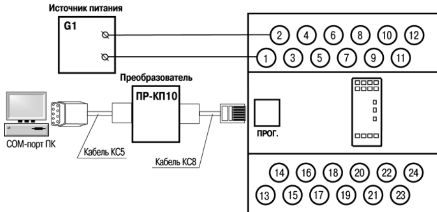
Рисунок Б.9 – Схема подключения PR110-х.8х.4х к ПК (через преобразователь PR-KP10), G1 – источник питания с номинальным напряжением, зависящим от исполнения прибора
