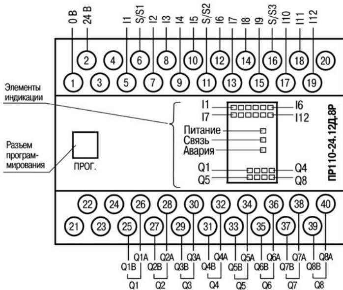
Рисунок Б.2 – Расположение контактов и элементов индикации в приборе PR110-24.12Д.8Р
