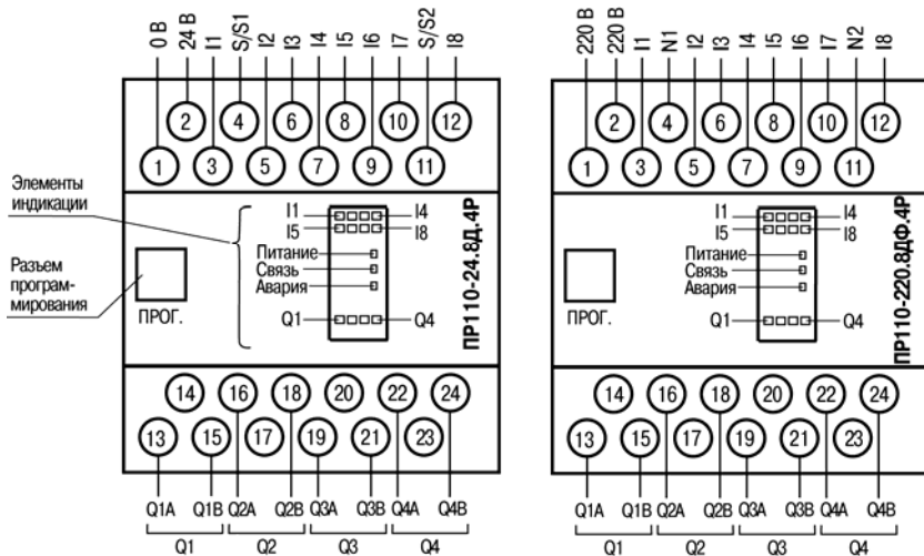
Рисунок Б.1 – Расположение контактов и элементов индикации в приборах ПР110
