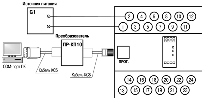
Рисунок Б.6 – Схема подключения PR110 к ПК (через преобразователь PR-KP10), G1 – источник питания с номинальным напряжением, зависящим от исполнения прибора
