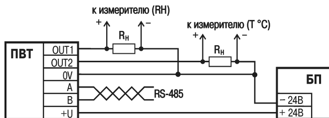
Рисунок 5.2 – Схема электрических соединений прибора
