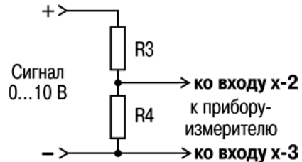
Рисунок 3.1 – Электрическая схема делителя ( R3=1800,0 Ом, R4=200,0 Ом)
