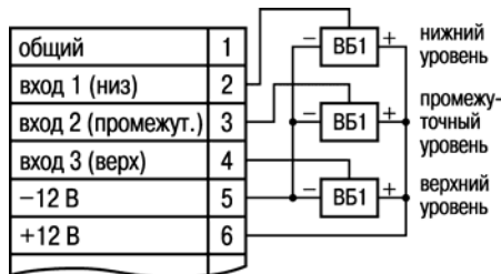
Рисунок Б.3 – Схема подключения емкостных переключателей
