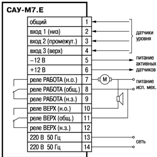
Рисунок Б.1 – Общая схема подключения САУ-М7.Е
