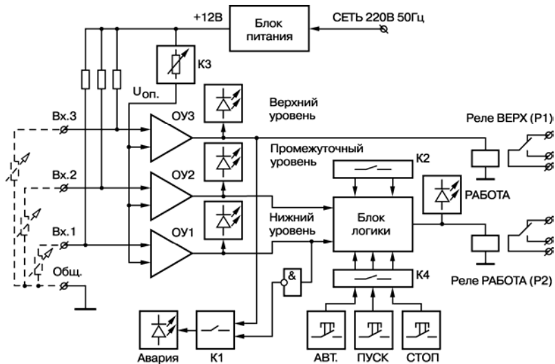
Рисунок 3.1 – Структурная схема прибора
