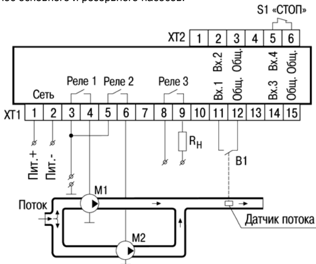
Рисунок В.6 – Схема подключения САУ-У-Н для выполнения алгоритма 11 М1 и М2 – насосы; Rн – сигнализатор аварии или дополнительный насос; B1 – датчик потока
