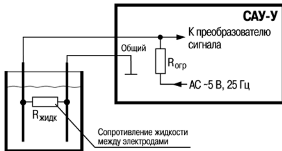
Рисунок 3.6 – Схема подключения кондуктометрического зонда
