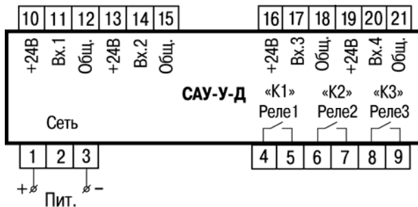
Рисунок Б.3 – Схема подключения САУ-У-Д
