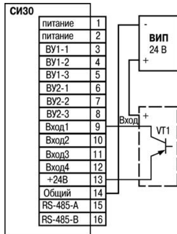
Рисунок Б.3 – Подключение к входу датчиков, имеющих на выходе транзистор р-п-р типа: а) активный датчик; б) пассивный датчик
