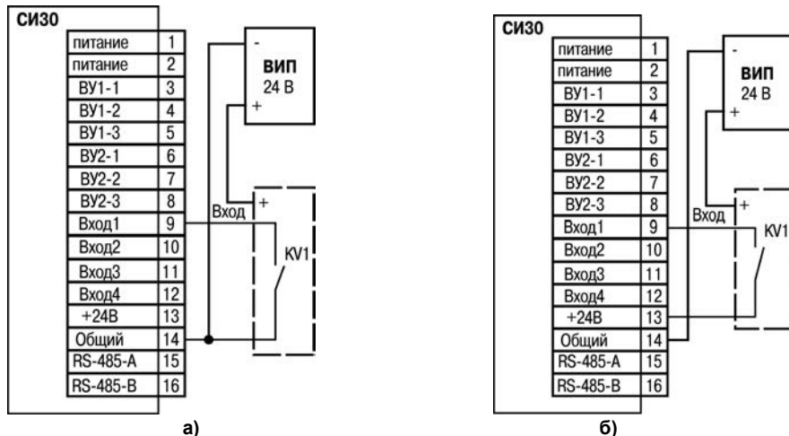
Рисунок Б.1 – Подключение к входу коммутационных устройств: а) при работе с n-p-n датчиками; б) при работе с р-n-p датчиками
