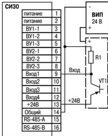
Рисунок Б.3 – Подключение к входу датчиков, имеющих на выходе транзистор р-п-р типа: а) активный датчик; б) пассивный датчик
