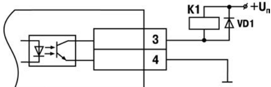
Рисунок Б.5 – Схема подключения нагрузки к ВУ типа К
