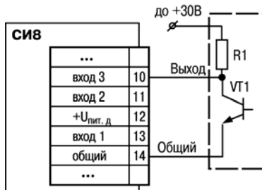
Рисунок Б.2 – Подключение датчиков с питанием от внешнего источника питания
