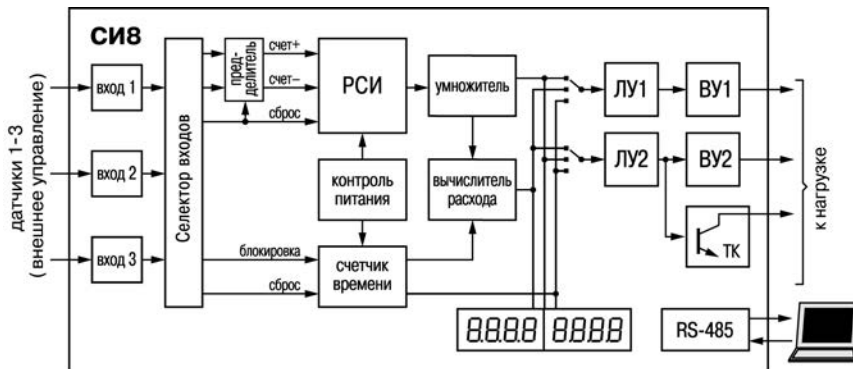
Рисунок 3.1 – Функциональная схема
