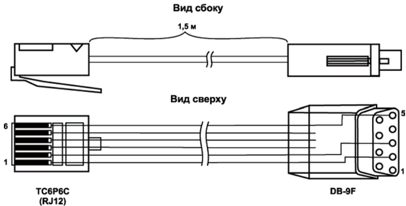
Рис. В.1. Схема распайки кабеля ПЛК-панель
