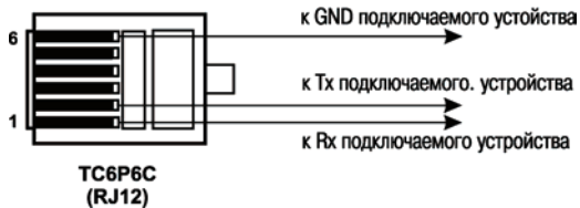
Рис. В.2. Схема распайки соединительного кабеля для подключения к порту RS-232 панели СМ1 1
