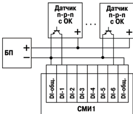
Рис Б.3. Схема подключения датчиков п-р-п типа с общим коллектором
