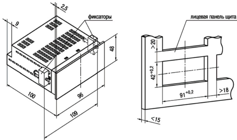
Рис А. 1 Габаритные и установочные размеры
