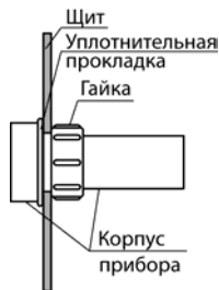
Рисунок 5.1 – Монтаж прибора в щит
