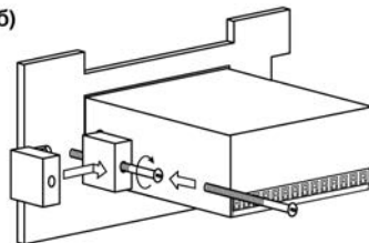
Рисунок 5.1 - Монтаж прибора щитового крепления
