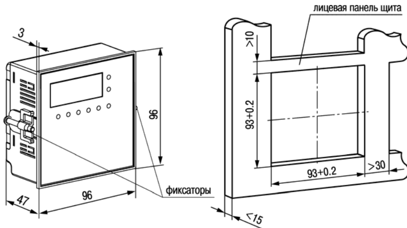
Рисунок А.1 – Габаритный и установочный чертежи корпуса прибора
