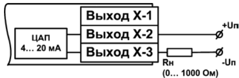
Рисунок Б.7 – Схема подключения нагрузки к ВУ типа И
