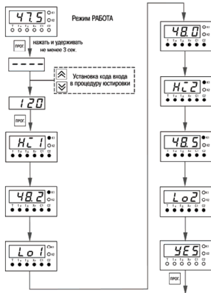
Рис. Ж.2. Последовательность запуска и индикации АНР для ТРМ10-Щ1.Р
